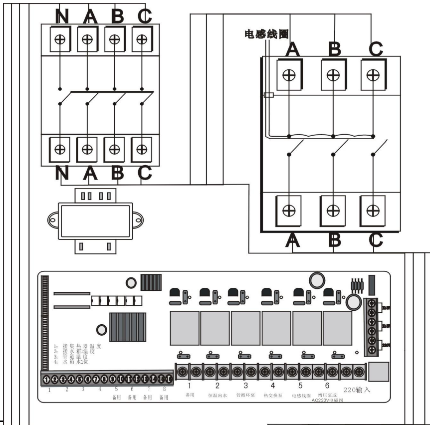
工程柜原理
